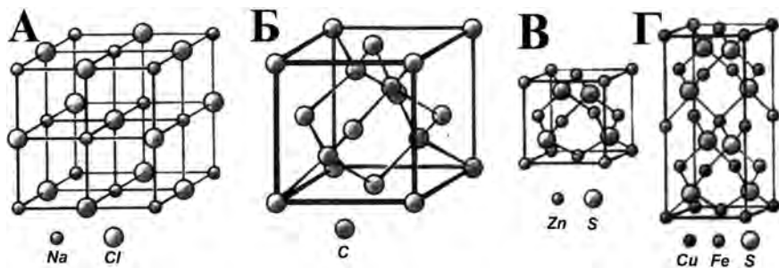
Рис. 1.3-2. Матричная структура кристаллических решёток кристаллов каменной соли (А), алмаза (Б), сфалерита (В) и халькопирита (Г).
